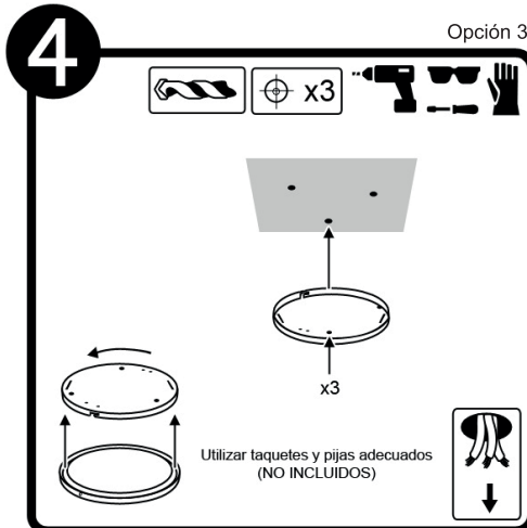
Option 3 Use proper anchors and screws (NOT INCLUDED) Utilisez des chevilles et des vis appropriées (NON INCLUSES)
