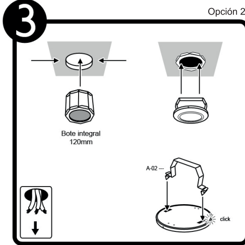
Option 2 Integral container 120mm-Pot intégré de 120mm
