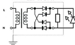
DIAGRAMA ELÉCTRICO: LED de 24 W
